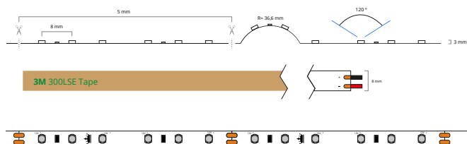
IP20 24V
